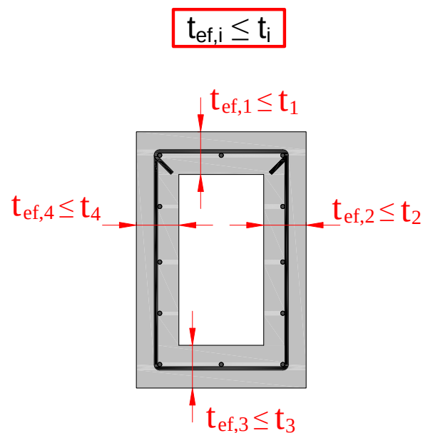
sandučasti presek
