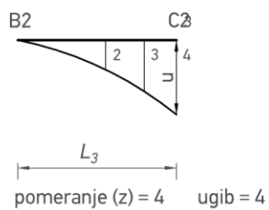
(e) Konzola B2 - C2
