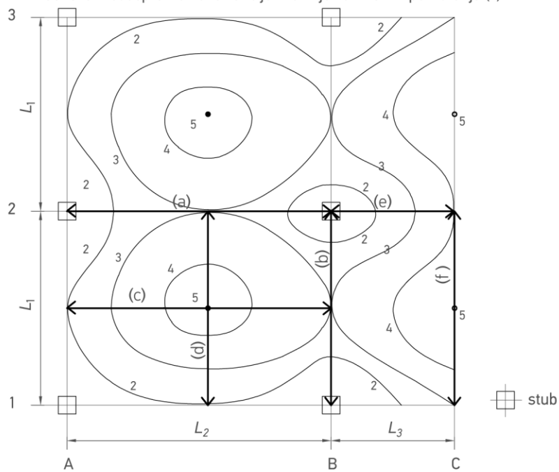
(a) Linija oslanjanja A2 - B2
