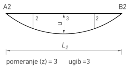
(a) Linija oslanjanja A2 - B2
