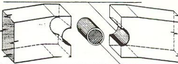
ČELIČNI CILINDAR NAPUNJEN BETONOM
